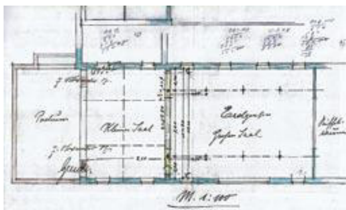
Abb. 8 Erdgeschossgrundriss von 1907 (Ausschnitt), Comesstraße 42 Repro aus: Bauakte der Stadt Brühl
